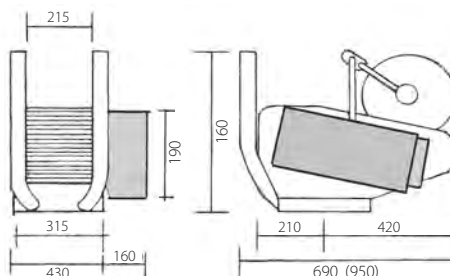
El-drevet garnspil. Idél til mindre både / Electrically driven nethauler. Ideal for smaller boats.
