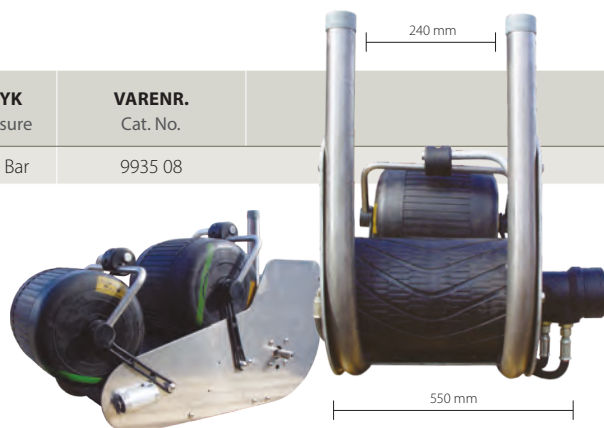
El-drevet garnspil. Idél til mindre både / Electrically driven nethauler. Ideal for smaller boats.
