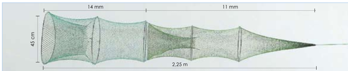
80 mailles // haut. 45 cm // 5 anneaux // filet noué vert.
