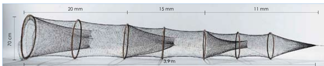
125 mailles // haut. 80 cm // 7 anneaux // filets noué noir.
