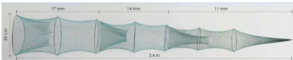
80 mailles // haut. 55 cm // 7 anneaux // filetsans noeuds vert.
